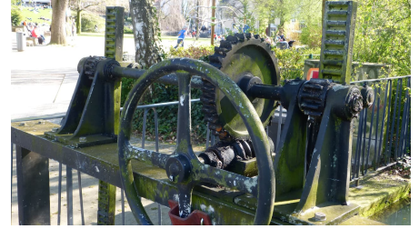
Wehr beim Funktionsmodell der Wasserkunst - © Karl Heinz Schäfer, Tourist Information Paderborn / Verkehrsverein Paderborn e.V.
