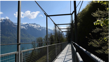
Hängebrücke Unterweidligraben ob Ebligen, zwischen Oberried und Brienz - © Christian Mathyer, Interlaken Tourismus
